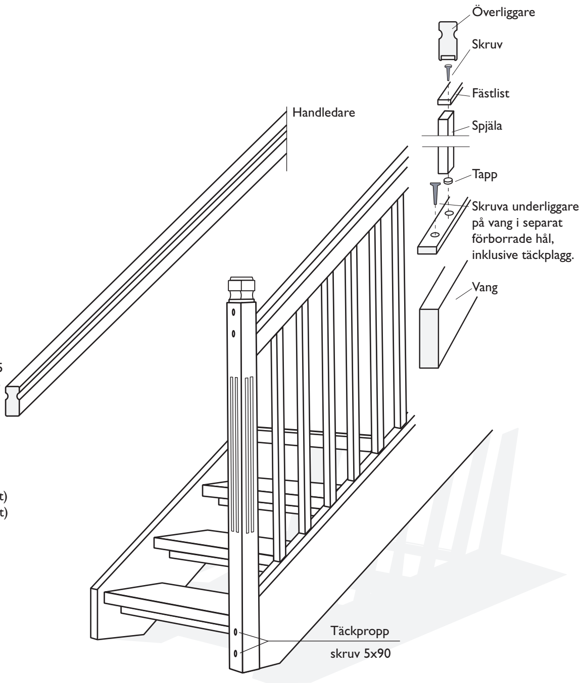
Underliggare på vång 30x45 Underliggare på golv 30x55
